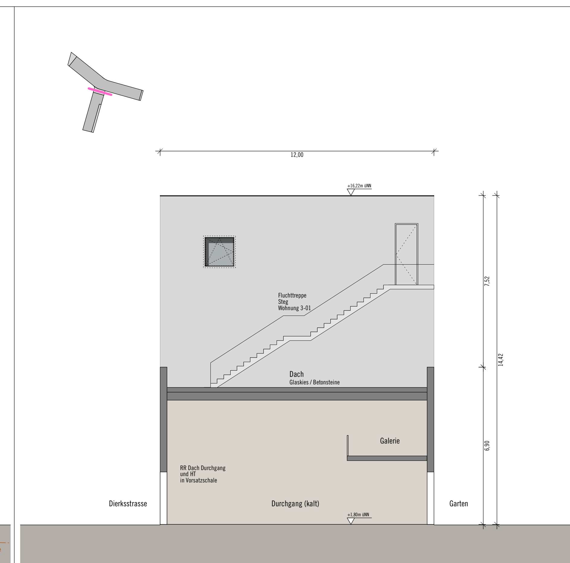
Ansicht 8 Nordseite / BT Steg
